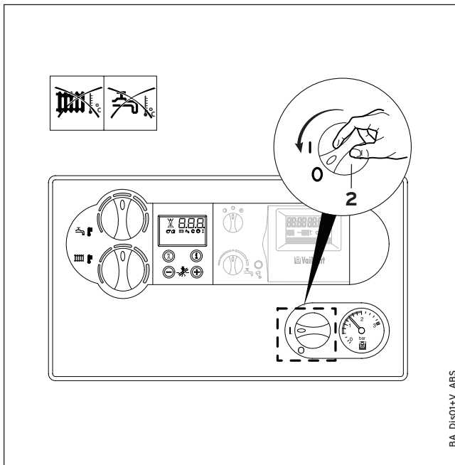
Afb. B.17: Volledig uit bedrijf nemen
