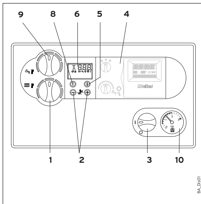
Afb. B.1: Bedienelementen
