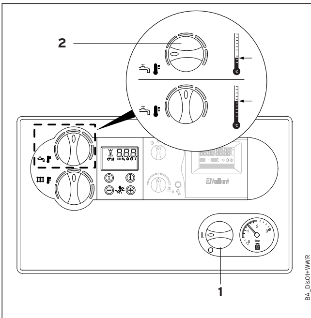
Afb. B.8: Warmwaterbereiding met een solotoestel
