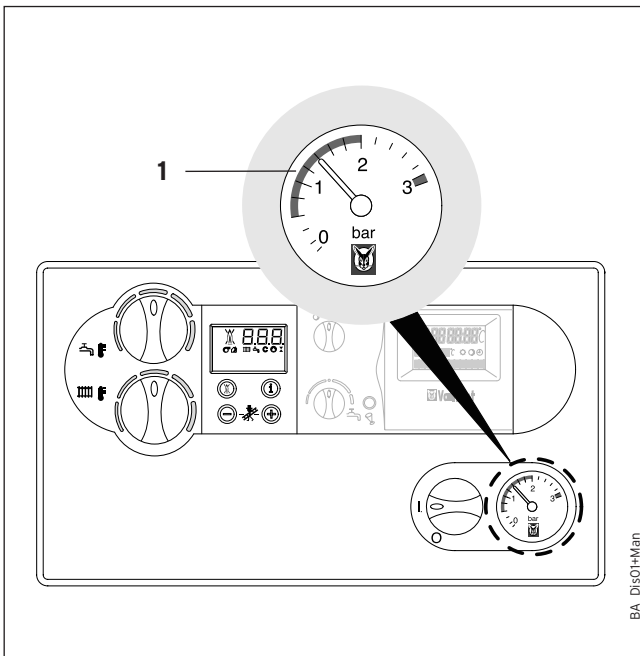
Afb. B.18: Toestel/cv-installatie vullen
