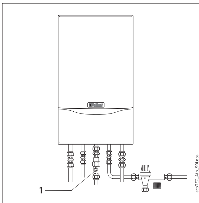
Afb. S.1: Gasstopkraan sluiten
