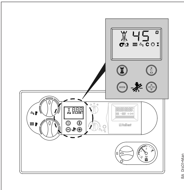
Afb. B.2: Display van het diagnosesysteem
