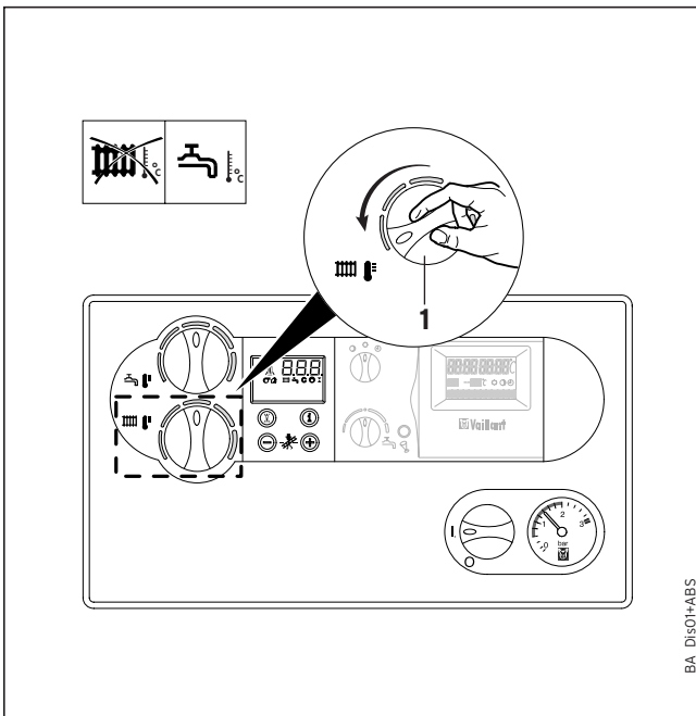
Afb. B.16: Verwarming uitschakelen (zomerbedrijf)
